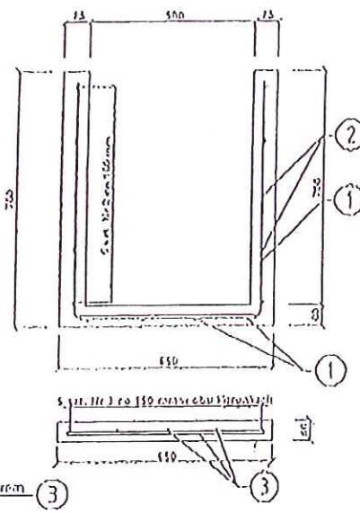
PRZEKRÓJ A-A
